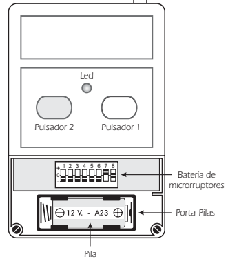
Caja abierta, sin tapa frontal.
